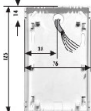
Základná doska senzora
